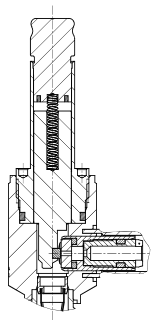
EX2 剖面图
