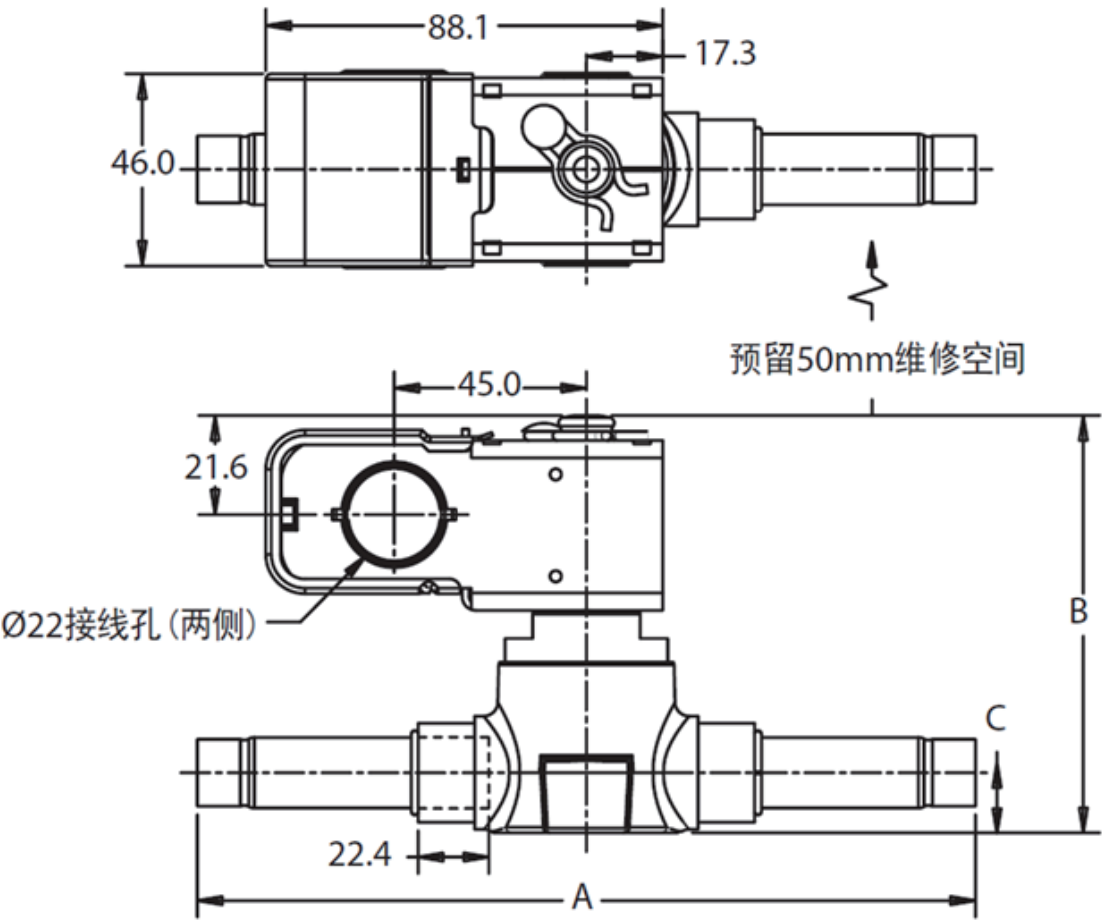
200RB 7系列和200RB 9系列的外形尺寸（mm）
