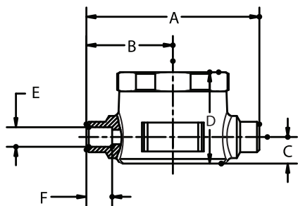
"SS" 型 ODFxODF
