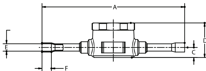
“TT”型
