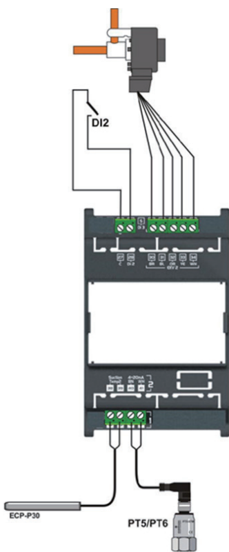
EXD-HP2 （上部板）
