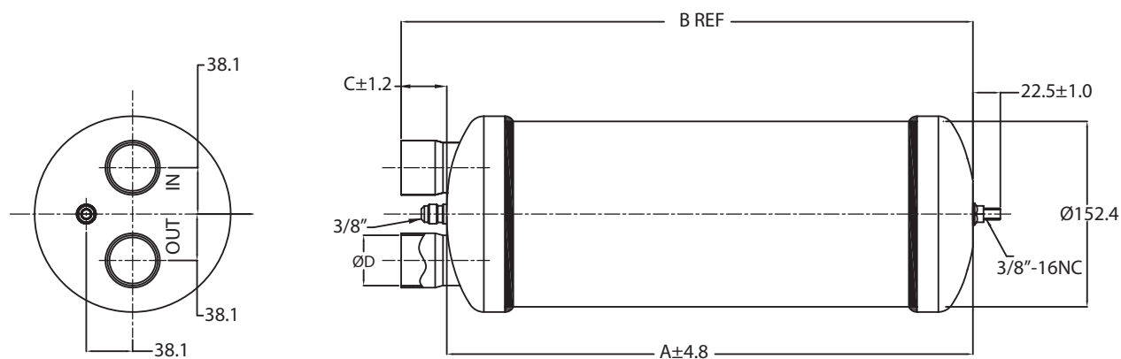
6 英寸油分离器外形尺寸图（单位：mm）
